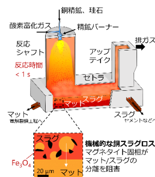
銅精鉱を酸化反応させる自溶炉の模式図
