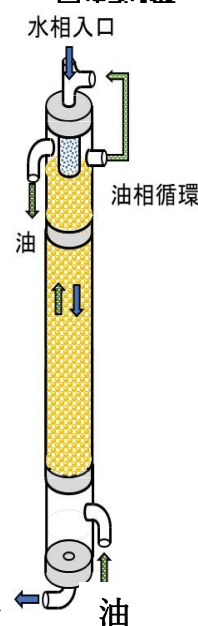
HIME カラム模式図
