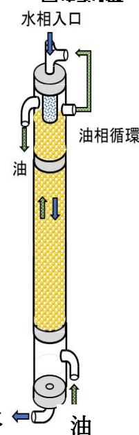
HIME カラム模式図
